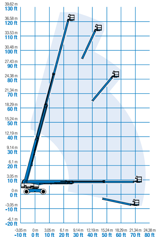
Courbe de travail S-125
